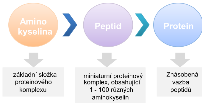
Struktura peptidu
